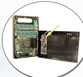
Carte réseau DL-NET Ajouté au boîtier du DL-10
